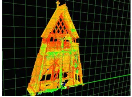
Klokkestabel, Borgund stavkirke, Fugro a/s 2004.
