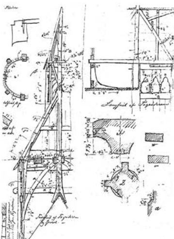
Nes stavkirke. Opmålingsskitser af G.A. Bull 1855.
