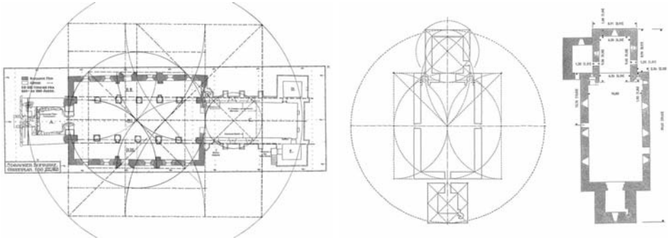
T.v.Stavanger Domkirke. Plan. T.h. Vaernes kirke. Plan.
